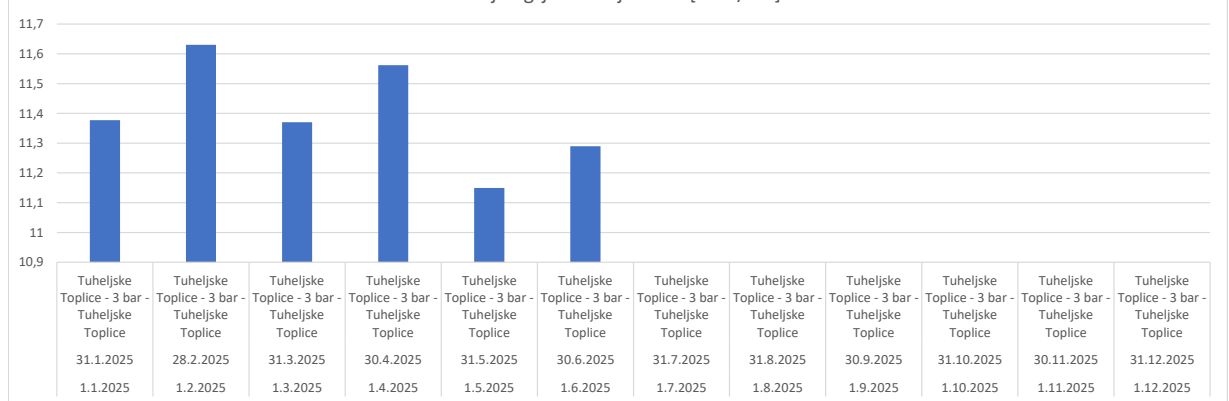
Gonja ogrjevna vrijednost [kWh/m3]
